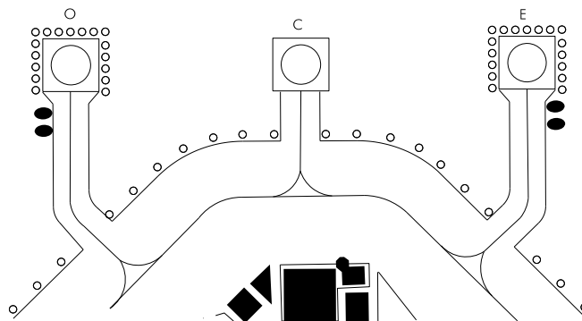
SGL & LGT FATO & TLOF
