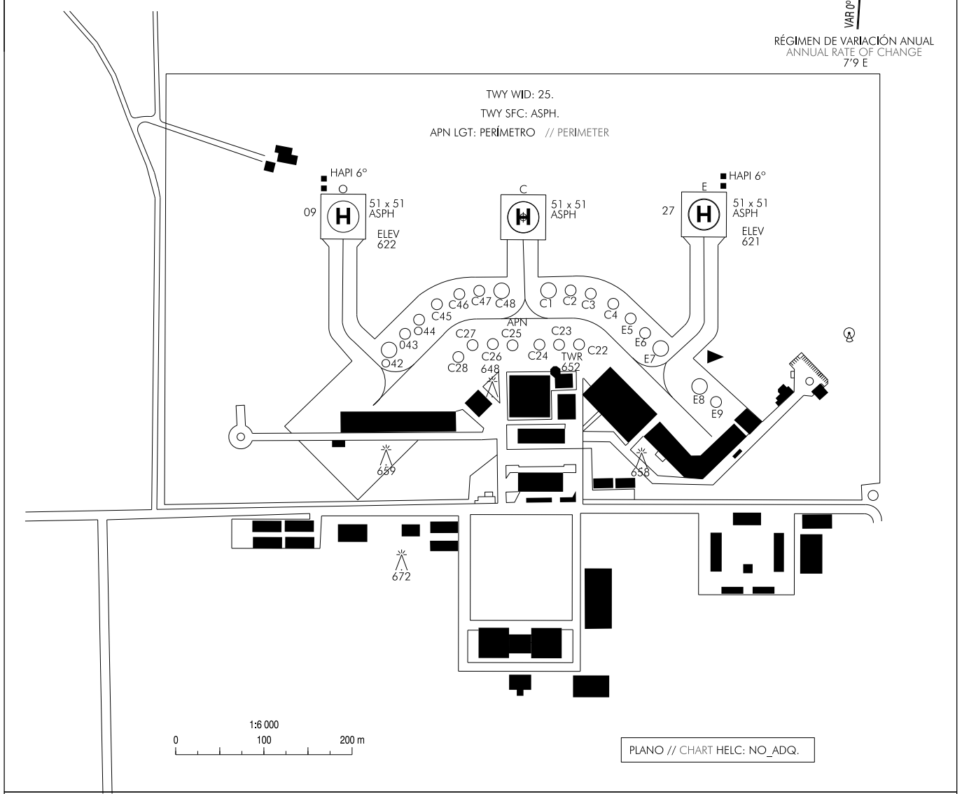
SGL & LGT FATO & TLOF
