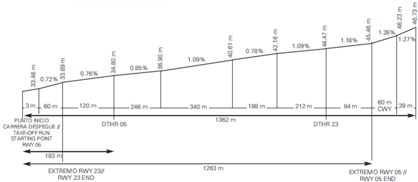
Perfil: RWY 05
