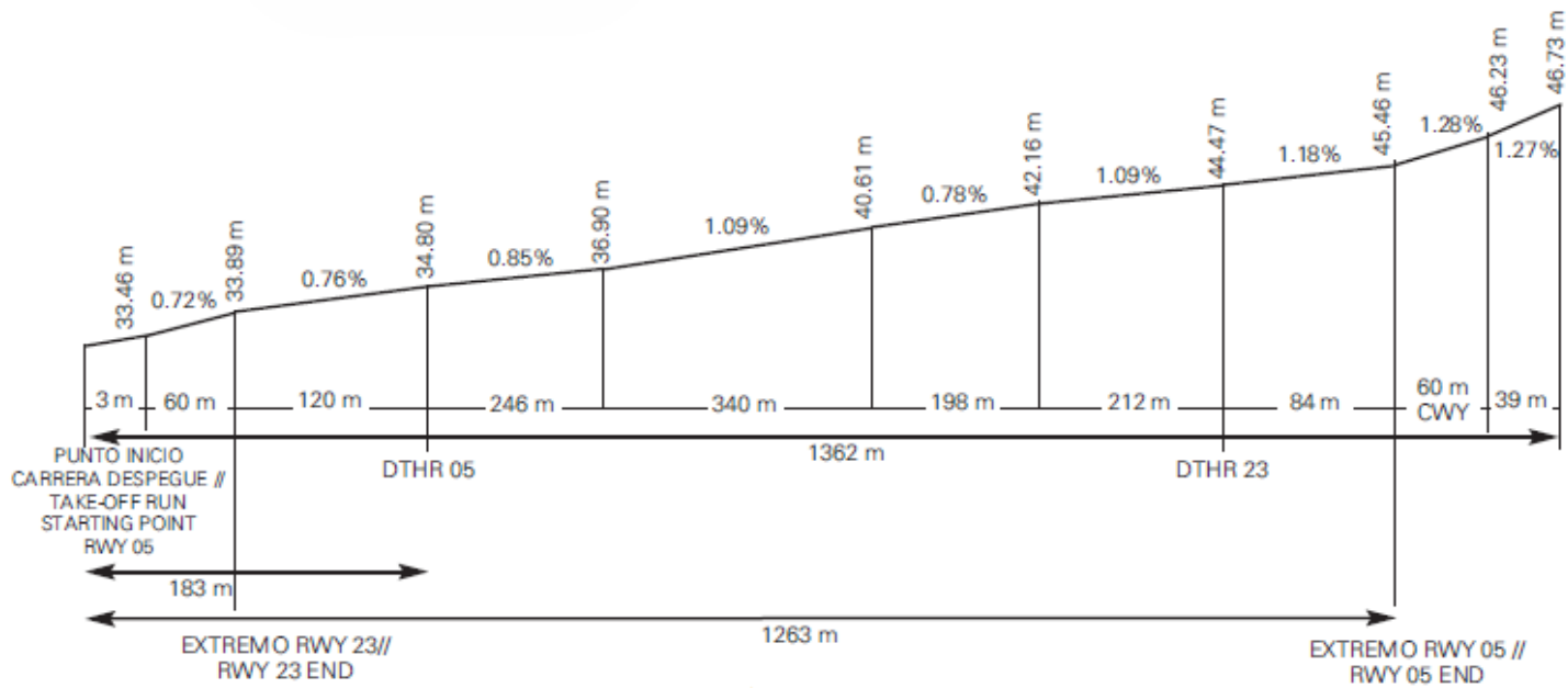
Perfil: RWY 05
