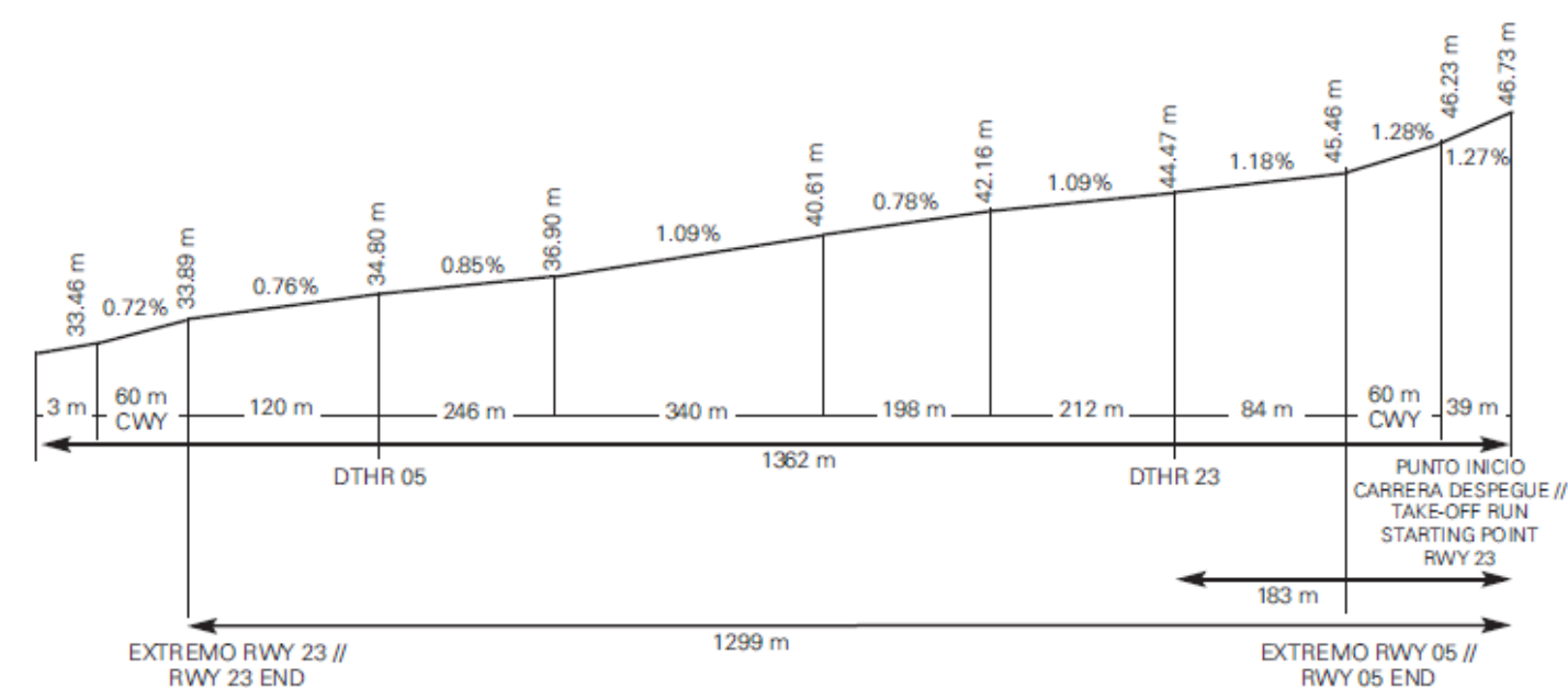
Perfil: RWY 23
