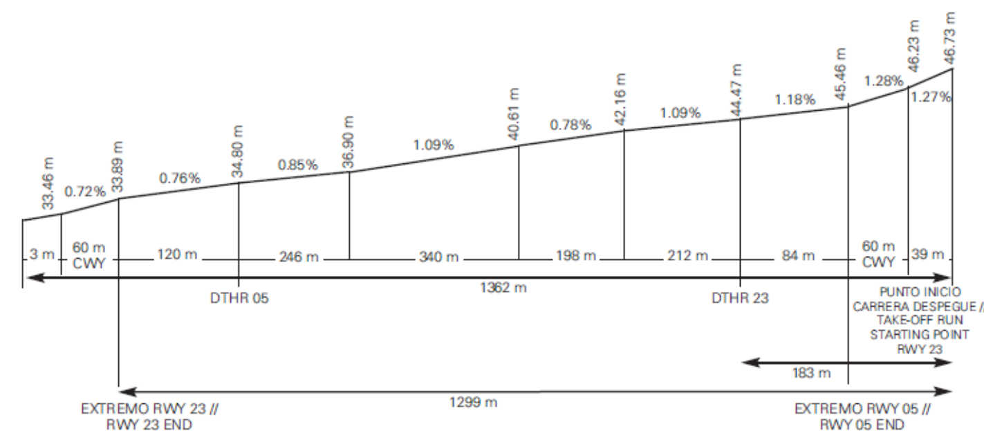
Perfil: RWY 23
