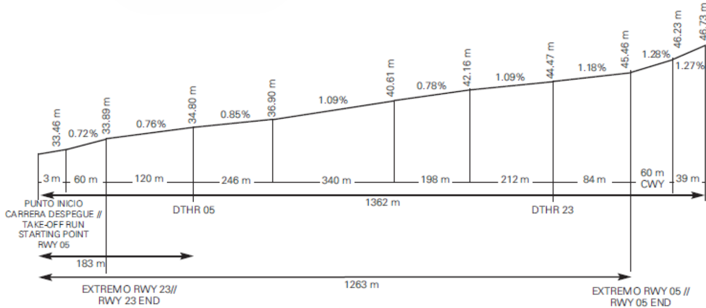
Perfil: RWY 05
